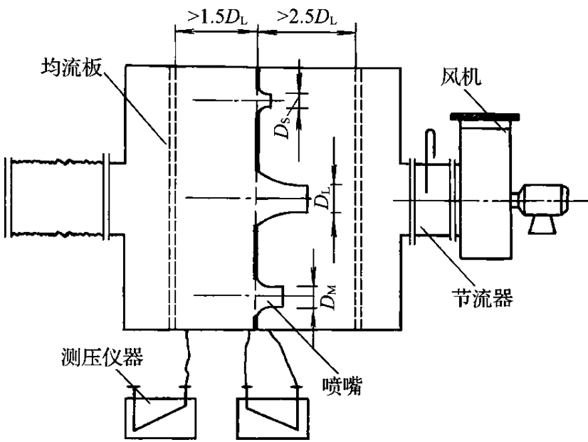
图 C. 2. 7-4 负压风室式漏风量测试装置
