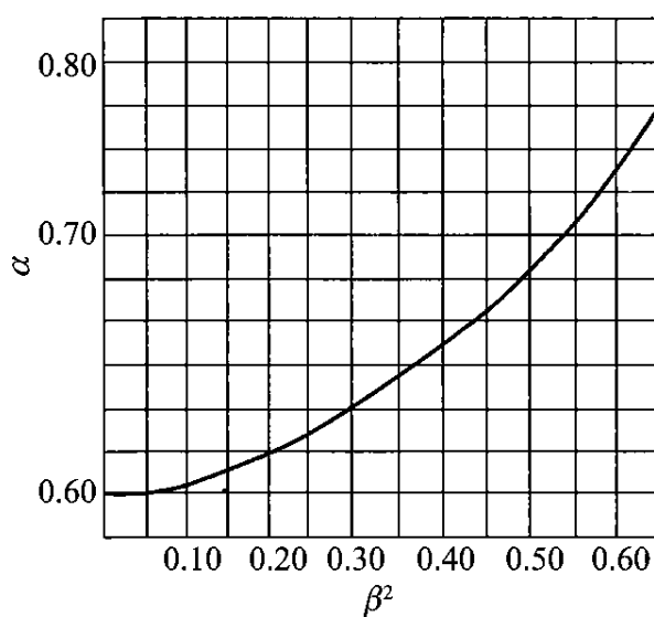
图 C. 2. 6-2 孔板流量系数图
