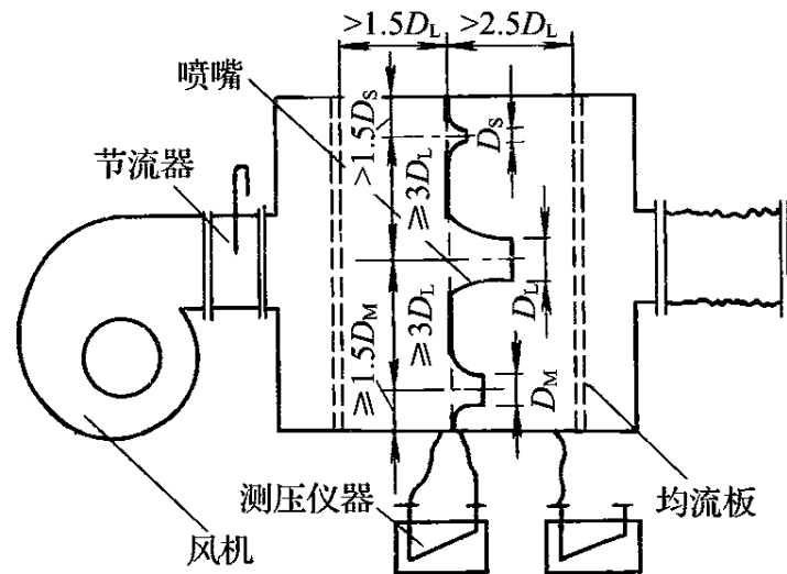
图 C. 2. 7-1 正压风室式漏风量测试装置
