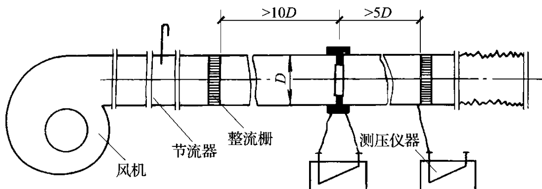
图 C.2.6-1 正压风管式漏风量测试装置
