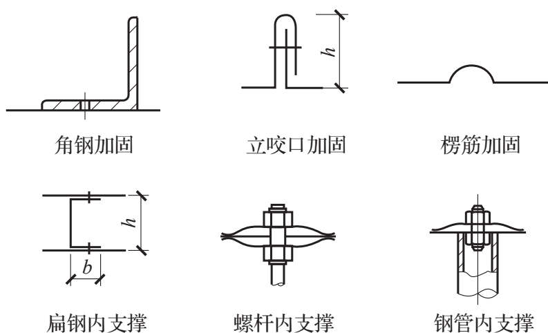
图 4.3.1 金属风管的加固形式
