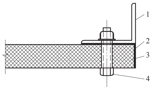
图 4.3.3 玻璃纤维复合风管角钢连接示意
