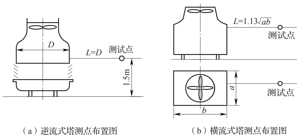
图 E. 6. 1-1 冷却塔测点布置图
