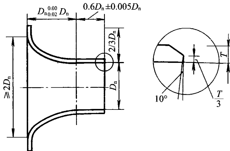
图 C. 2. 7-2 标准长颈喷嘴
