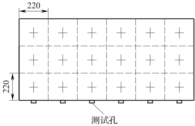
图 E. 1. 3-1 矩形风管测点布置示意
