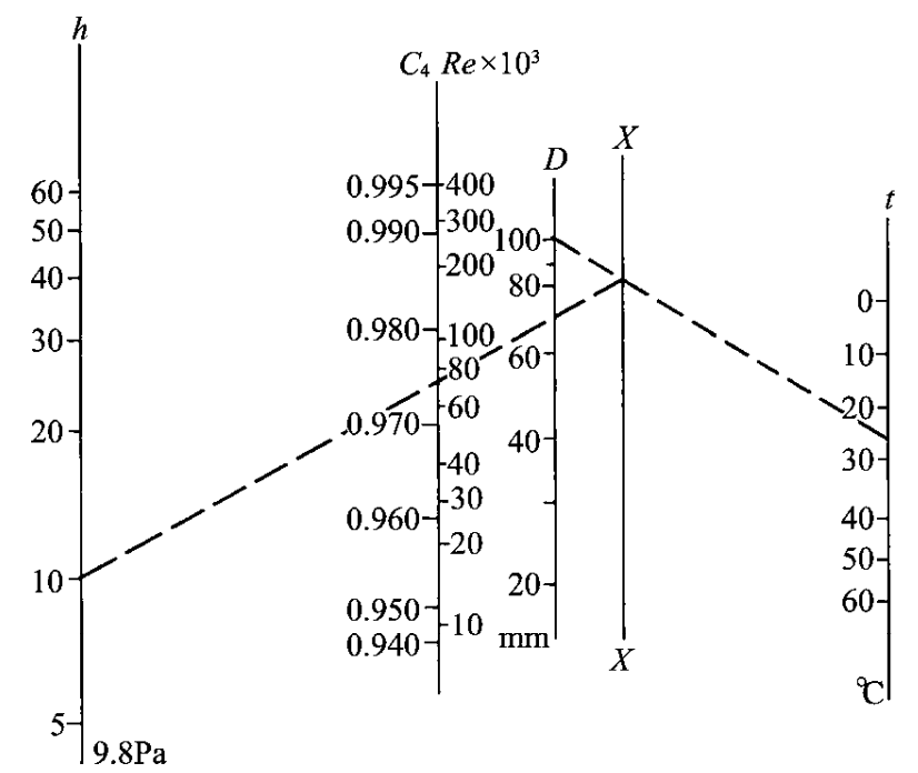
图 C. 2. 7-3 喷嘴流量系数推算图
