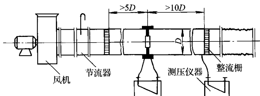
图 C.2.6-3 负压风管式漏风量测试装置
