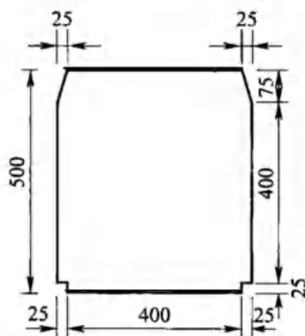
图 13 车行横通道的断面建筑限界(cm)
