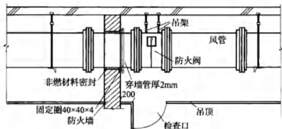
图 10 防火阀检修口设置示意图
