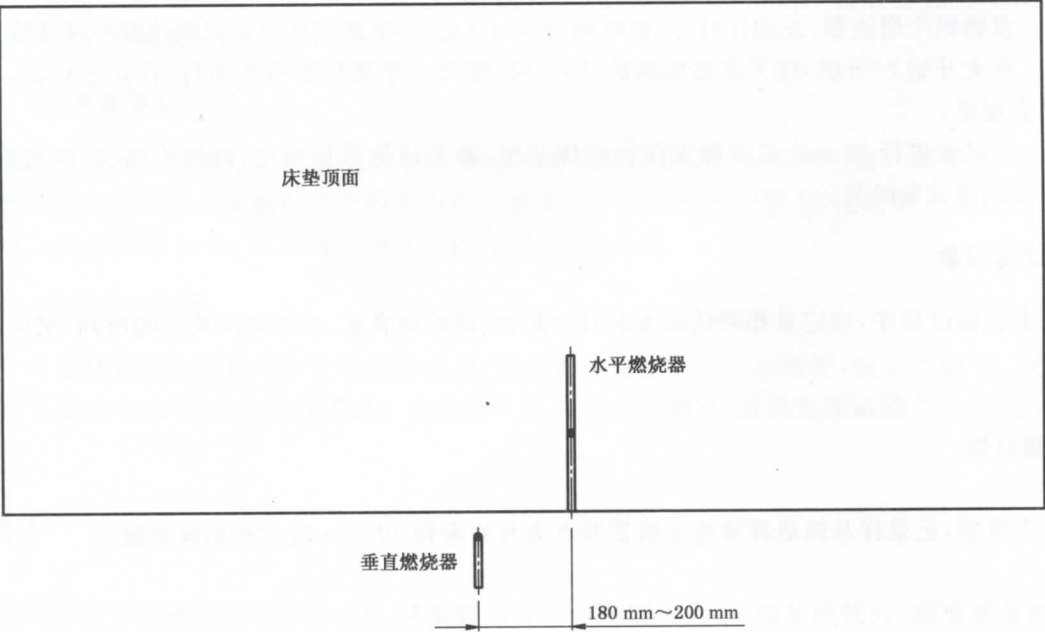
b) 俯视图
