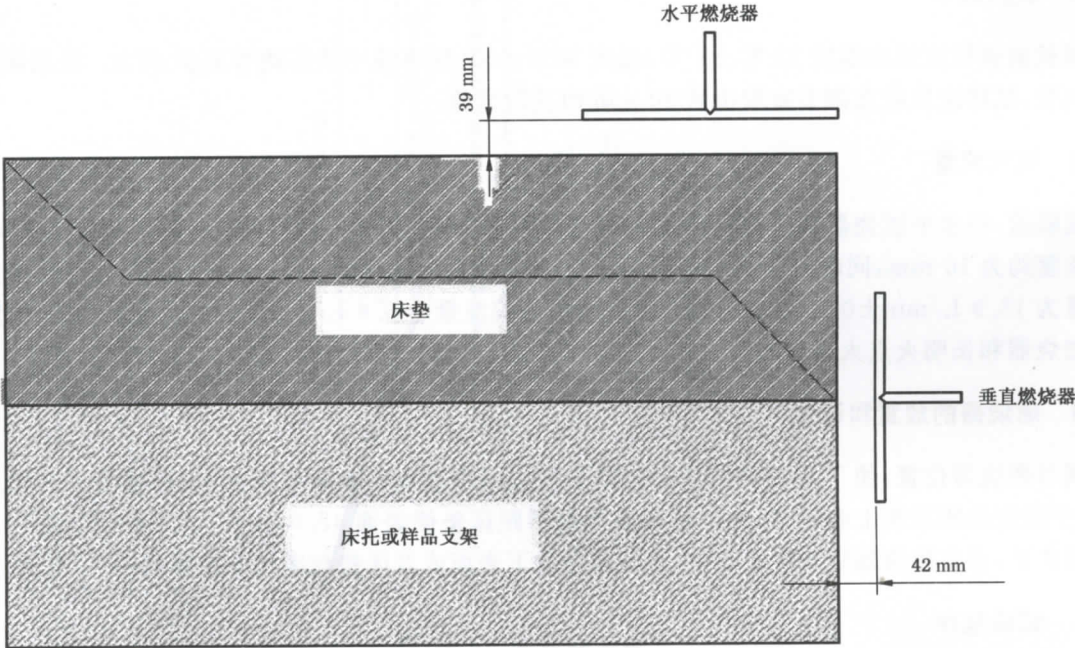
a) 侧视图
